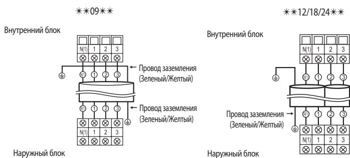
Внутренний блок
